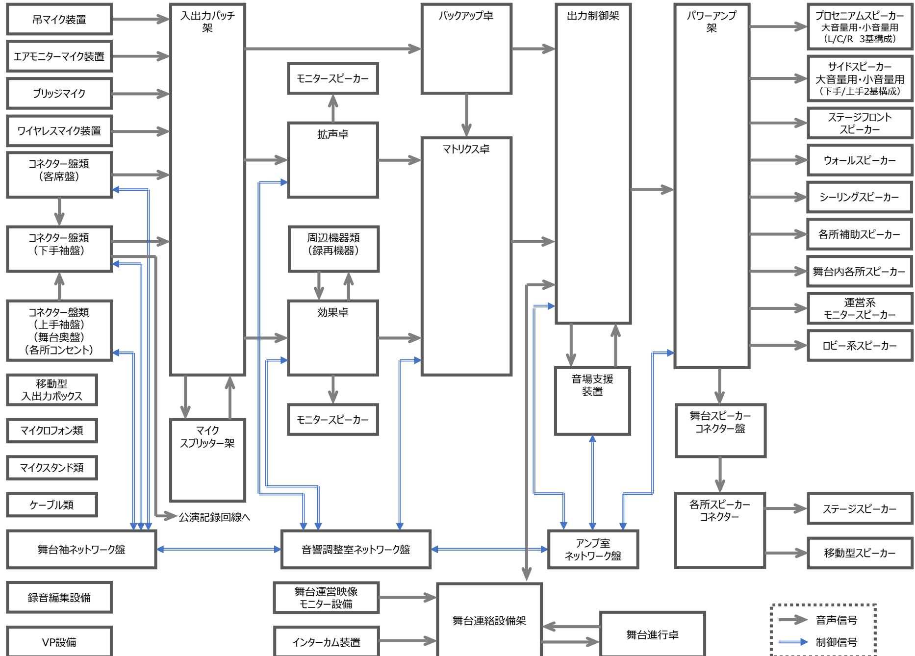
国立劇場 小劇場 舞台音響設備 ブロック系統図
