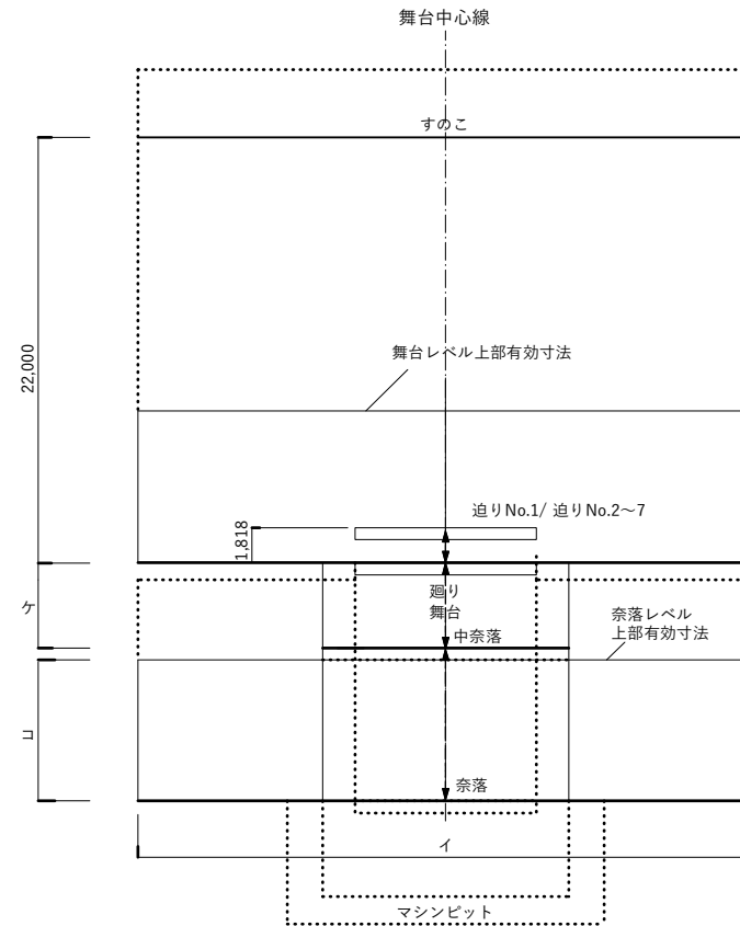
舞台断面図
