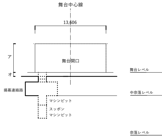
客席断面図
